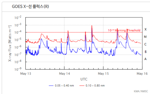
태양 엑스선 플럭스
