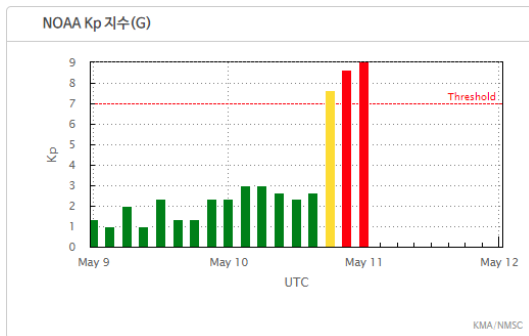
지구자기장 교란지수
