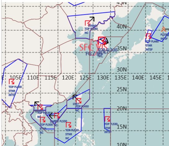
공역경보(SIGMET) 07.04. 15:00KST
