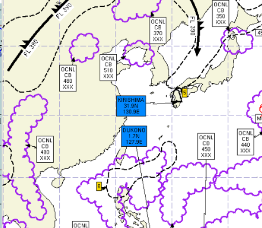
공역예보(SIGWX) 07.05. 03:00KST
